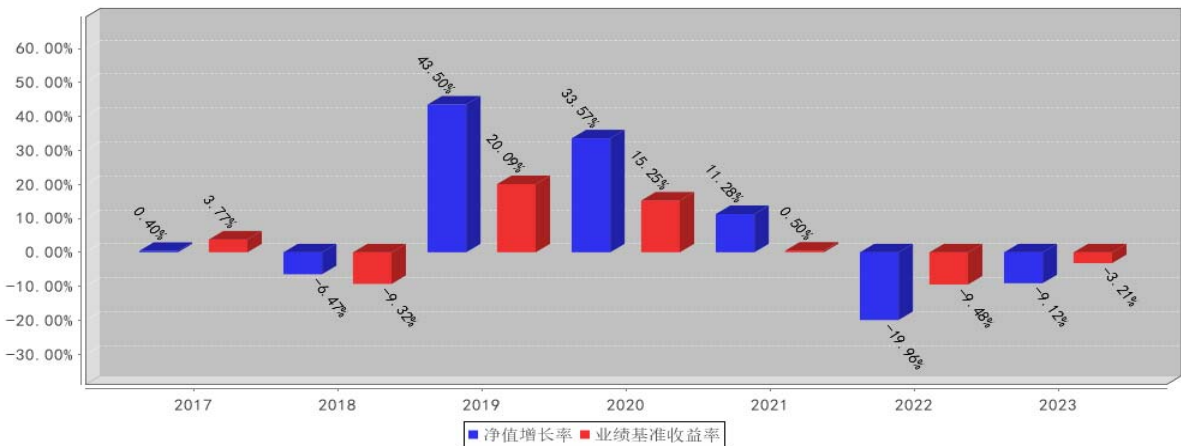
西部利得新润混合A基金每年净值增长率与同期业绩比较基准收益率的对比图（2023年12月31日）
